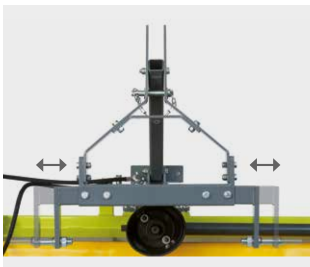
Attacco 3° punto Cat. 1 o 2 registrabile Adjustable 3-point linkage Cat. 1 or 2 Verstellbarer 3-Punkt Anbau Kat. 1 oder 2 Attelage réglable (2 positions)
